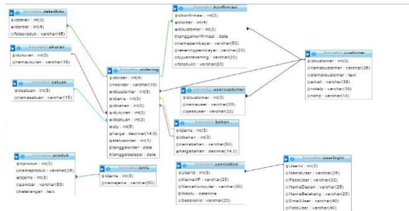
Gambar 3. Class Diagram Sistem yang berjalan
