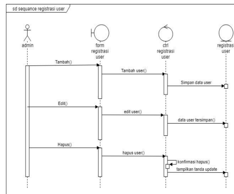
Gambar 4. Sequence Diagram sistem yang berjalan
